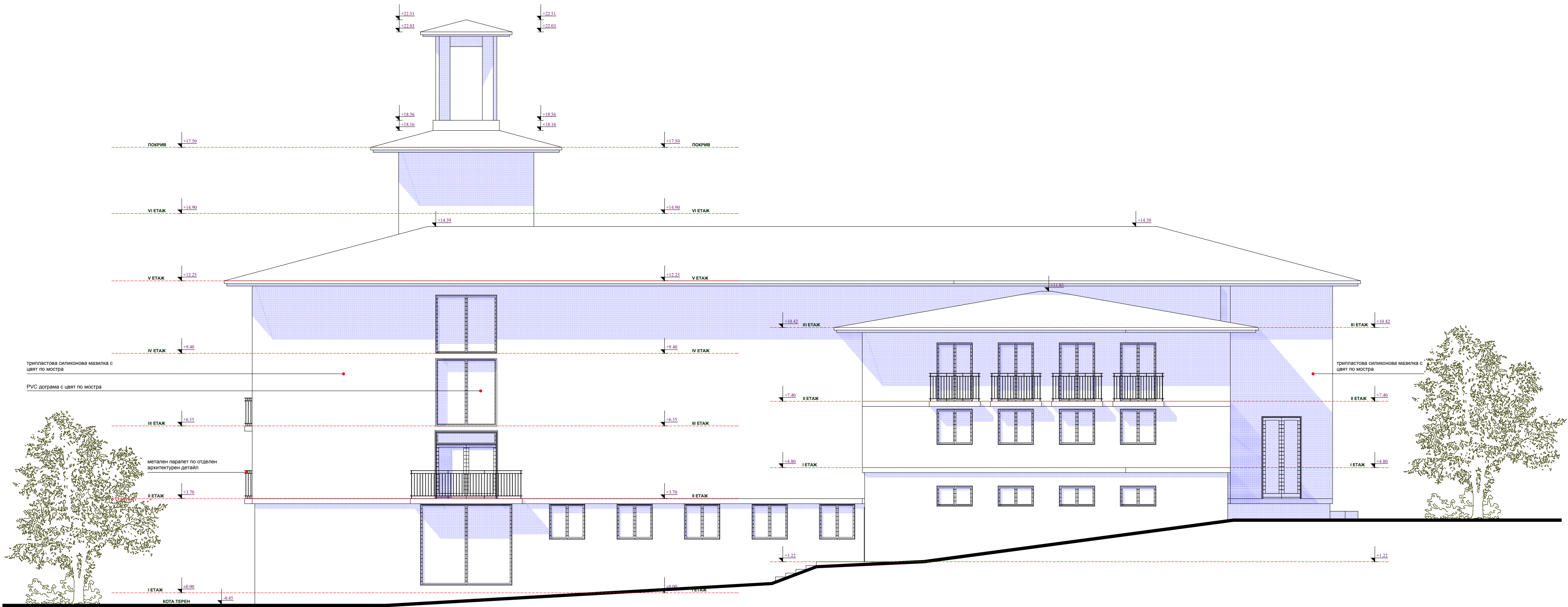
ФАСАДА ЮГОИЗТОК
